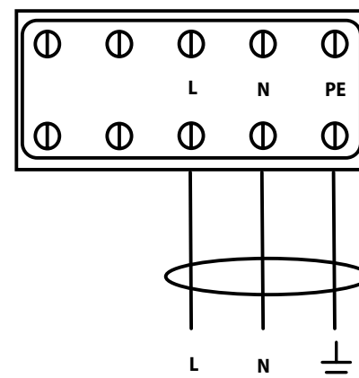
Joonis 3A – Toitekaabli ühendamine sisemise ventilaatori kiiruselülitiga varustatud seadmél. Seadme põhitoide.
