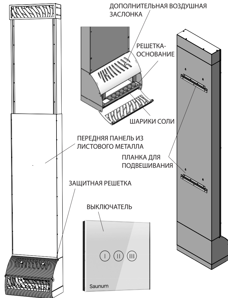
Рис. 2В – Детали устройства Saunum BASE S.
