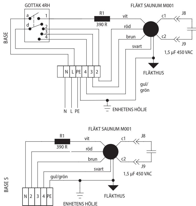
Figur 5 – Kopplingsschema för enhet utan reglage, med belysning.
