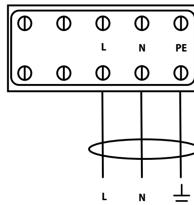
Figur 3A – Anslutning av strömkabel för en enhet med invändigt reglage för fläkthastighet. Huvudström till enheten.
