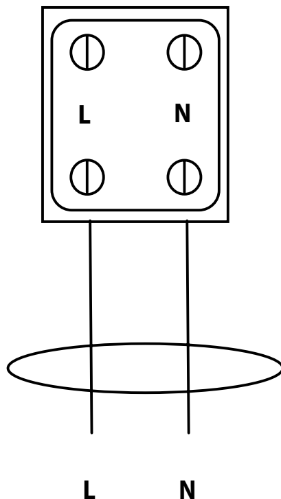
Kuva 3 – Syöttökaapelin liittäminen sisäisen tuulettimen nopeusvalitsimilla varustetussa laitteessa.
