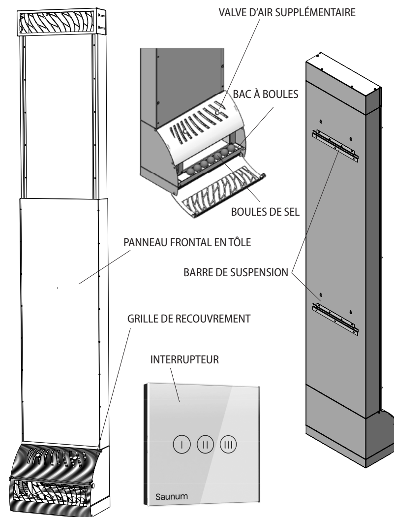
Figure 2B – Composants du modèle Saunum BASE S.
