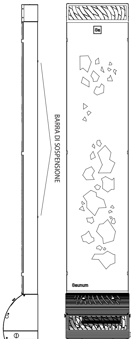
Figura 1E – Installazione consigliata del modello Saunum BASE / BASE Short con una barra di sospensione.
