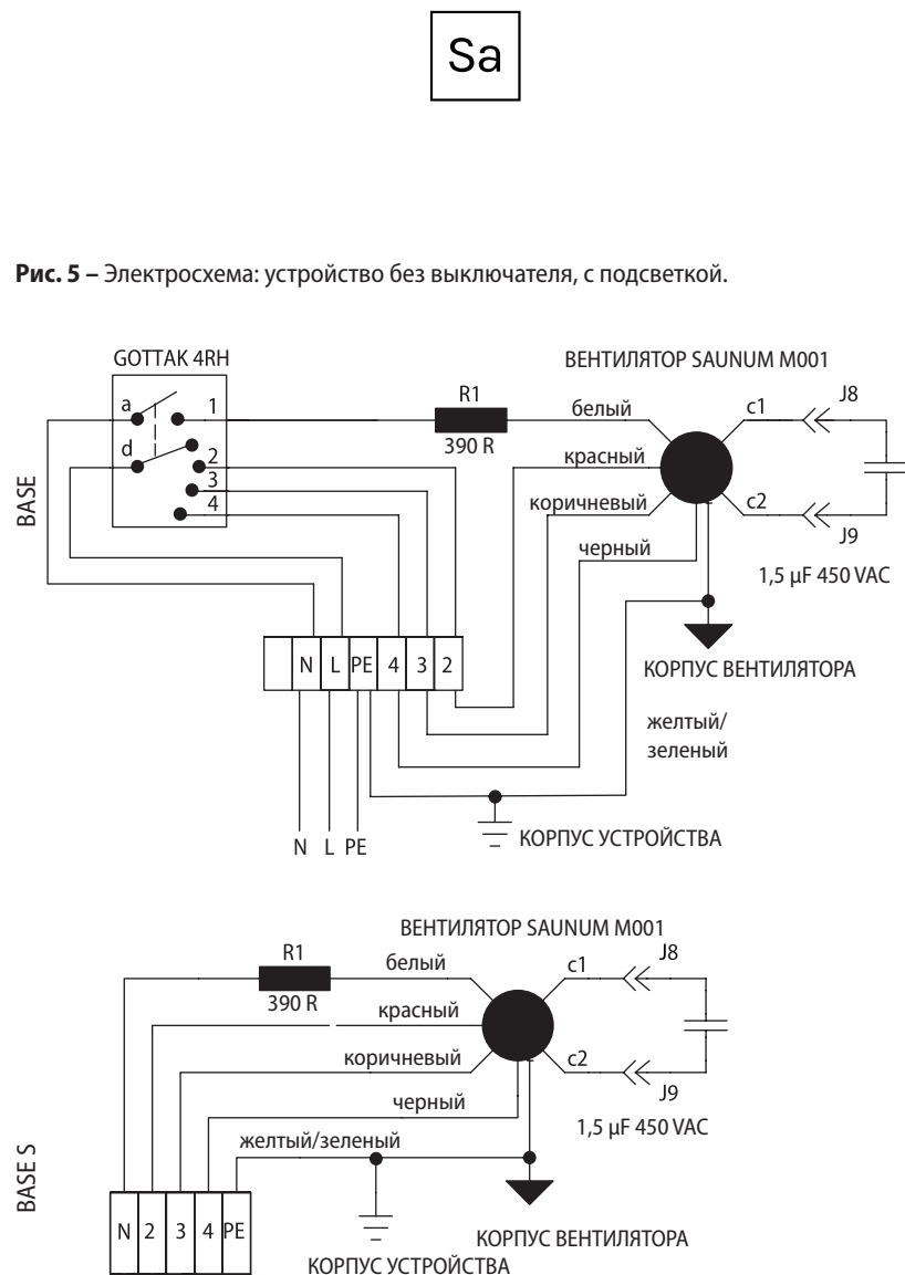
ПИТАНИЕ/СКОРОСТЬ ВХОДНАЯ КЛЕММА ПИТАНИЯ ВЕНТИЛЯТОРА 230VAC ВНИМАНИЕ! РАЗРЕШЕНО ПОДКЛЮЧАТЬ ТОЛЬКО ЧЕРЕЗ УСТРОЙСТВО ЗАЩИТНОЙ АВТОМАТИКИ!
