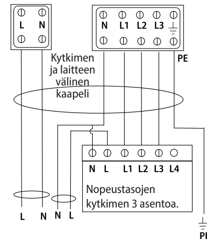
Kuva 4 – Syöttökaapelin liittäminen tuulettimen nopeuskytkimellä varustettuun laitteeseen.
