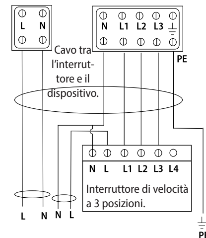
Figura 4 – Collegamento del cavo di alimentazione su un dispositivo dotato di interruttore esterno di velocità del ventilatore.
