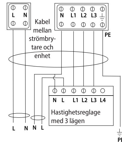
Figur 4 – Anslutning av strömkabel för en enhet med externt reglage för fläkthastighet.
