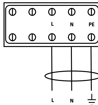
Kuva 3A – Syöttökaapelin liittäminen sisäisen tuulettimen nopeuskytkimellä varustetussa laitteessa. Laitteen perussyöttö.
