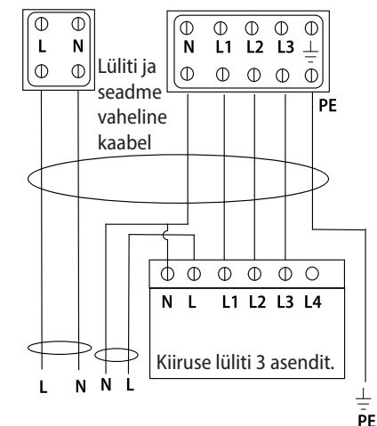
Joonis 4 – Toitekaabli ühendamine välise ventilaatori kiiruselülitiga varustatud seadmél.
