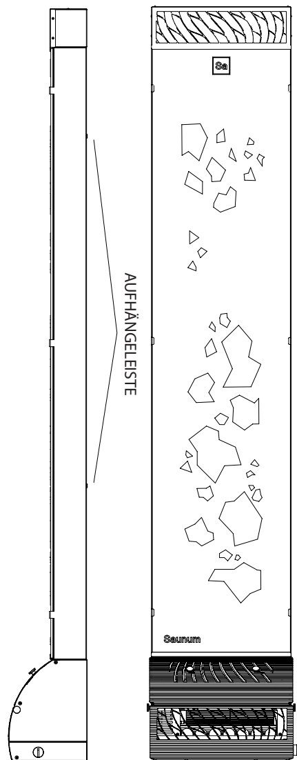
Abbildung 1E – Empfohlene Installation des Geräts des Modells Saunum BASE/ BASE Short mit Aufhängeleisten.
